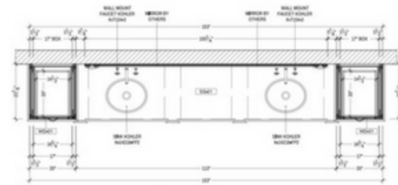
2 PLAN SECTION SCALE: 1/8"=1'-0"
