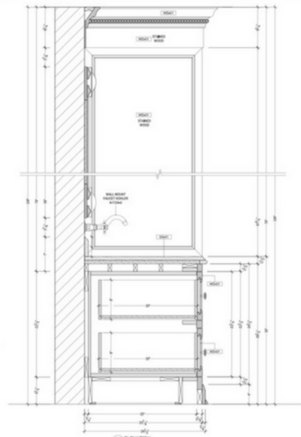
S3 ELEVATION SCALE: 1/8"=1'-0"
