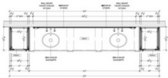
3 PLAN SECTION SCALE: 1/8"=1'-0"
