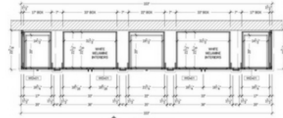
1 PLAN SECTION SCALE: 1/8"=1'-0"
